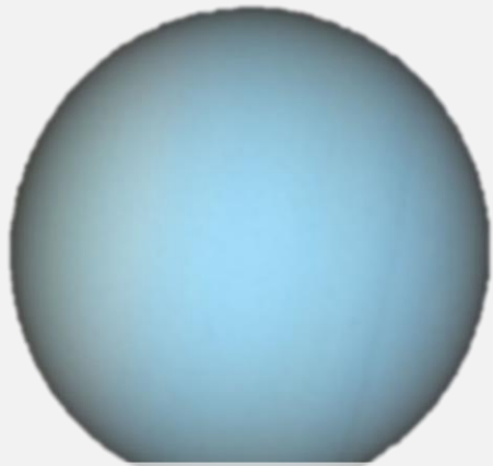
Uranus
